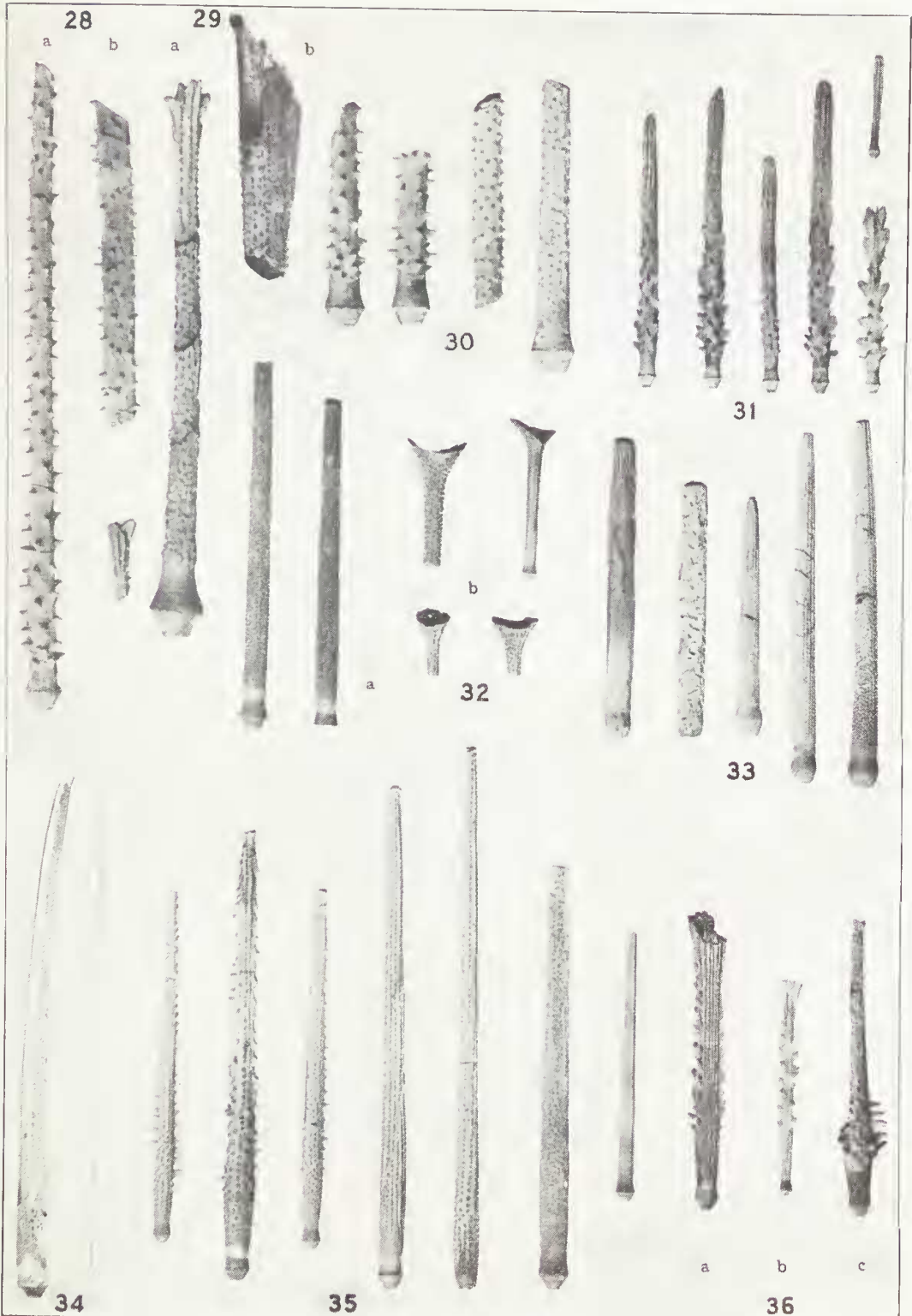
Cainozoic Cidaroids
